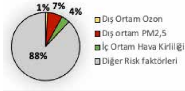
Şekil 2. Hava kirliliğine atfedilen küresel ölüm yüzdesi [10]
